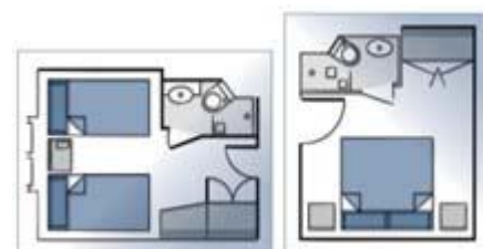
План кают
